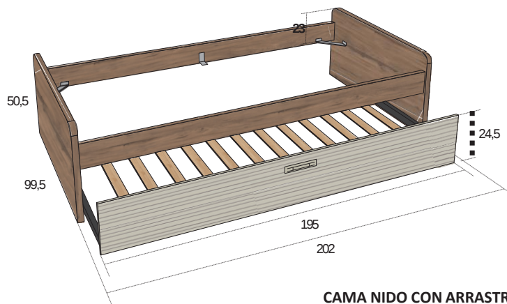
CAMA NIDO CON ARRASTRE
