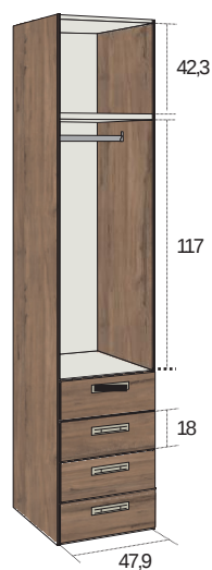
ARMARIO 1 PUERTA + 4 CAJONES 51cm. (240)
