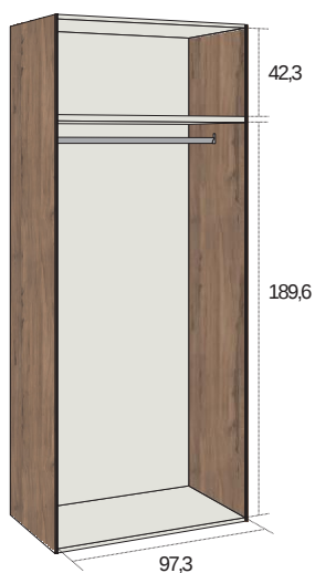
ARMARIO 2 PUERTAS 101cm. (240)
