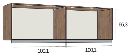
PUENTE 4 PUERTAS BATIENTES 205cm.
