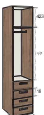
ARMARIO 1 PUERTA + 4 CAJONES 51cm. (240) Pino Coco Tirador "Lower" Gris Coco
